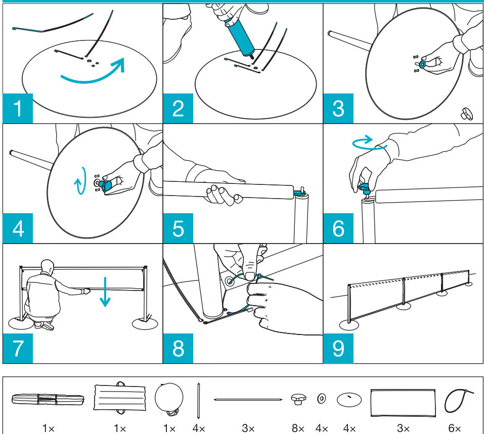
Zeichnung 2. Installationsreihenfolge von Werbehürde auf dem harten Boden (Satz Basis 11 + 2 Extras 12 )
