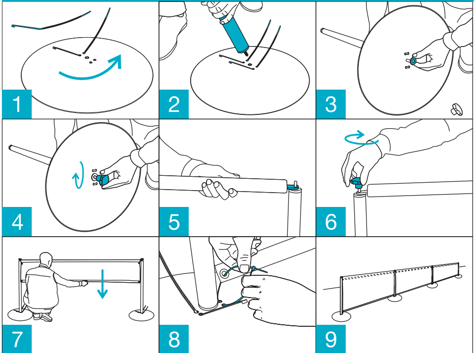
Rys. 2. Instrukcja montażu płotka na podłożu twardym w pomieszczeniu zamkniętym (zestaw baza 3 + 2 dostawki 4 )
