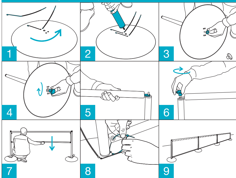
Obrázek 2: Postup montáže plotového pole na pevném podkladu (set základního modulu 3 + 2 rozšiřujících modulů 4 )
