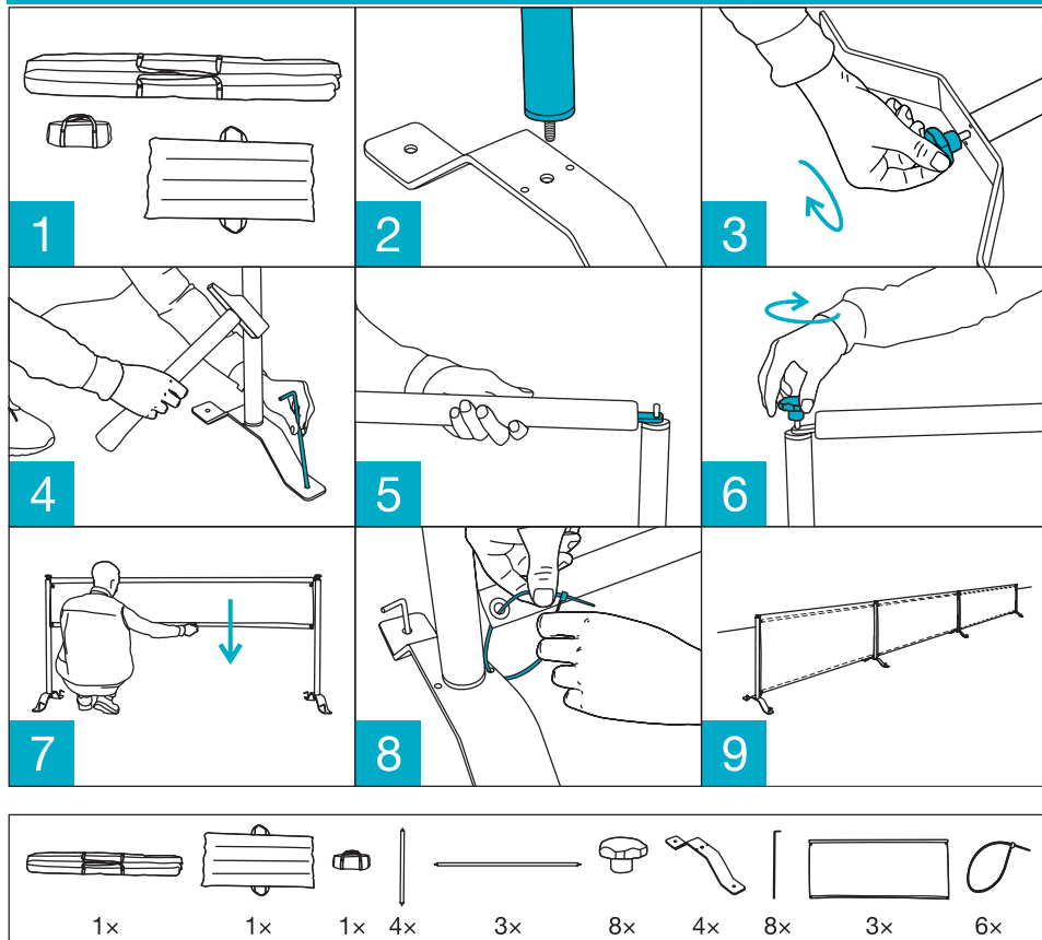
Rys. 1. Przebieg montażu na podłożu miękkim (zestaw baza 1 + 2 dostawki 2 )
