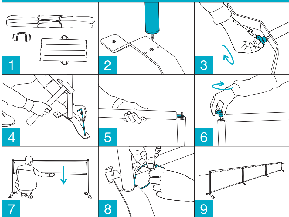
Obrázek 1. Postup montáže plotového pole na měkkém podkladu (set základního modulu 1 + 2 rozšiřujících modulů 2 )
